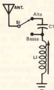
Fig. 2 - L'accoppiatore migliorato ha un commutatore ad una via e due posizioni che inserisce od esclude il condensatore C1 da 100 pF. L'accordo fine dell'antenna si fa regolando il nucleo di L1.
