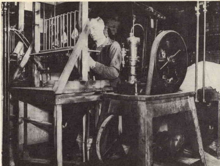
Ricostruzione di un sistema di pompe per lampade a filamento di carbone quale deve essere stato usato da Gerard Philips agli inizi. Questa ricostruzione venne fatta nel 1951 in occasione del 60° anniversario della Società; il sistema rimase in funzione parecchie settimane.
