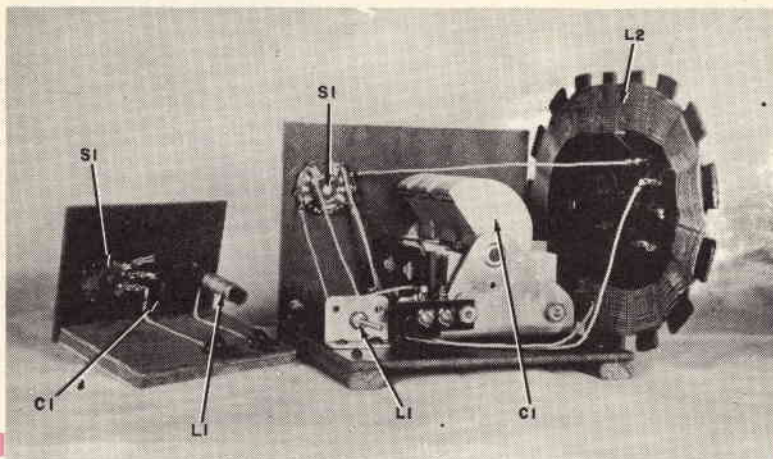
Fig. 2 - L'accoppiatore migliorato ha un commutatore ad una via e due posizioni che inserisce od esclude il condensatore C1 da 100 pF. L'accordo fine dell'antenna si fa regolando il nucleo di L1.
