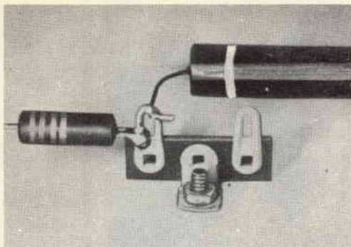
Il resistore con il terminale arrotolato (a sinistra) dovrà essere sacrificato: i terminali sono troppo corti e la connessione meccanica troppo stretta. Fate il confronto con il condensatore a destra.
