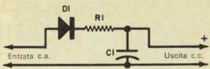
Fig. 3 - Per limitare le sovracorrenti si è inserito il resistore R1 tra il raddrizzatore a mezz'onda DI ed il condensatore di filtro C1.
