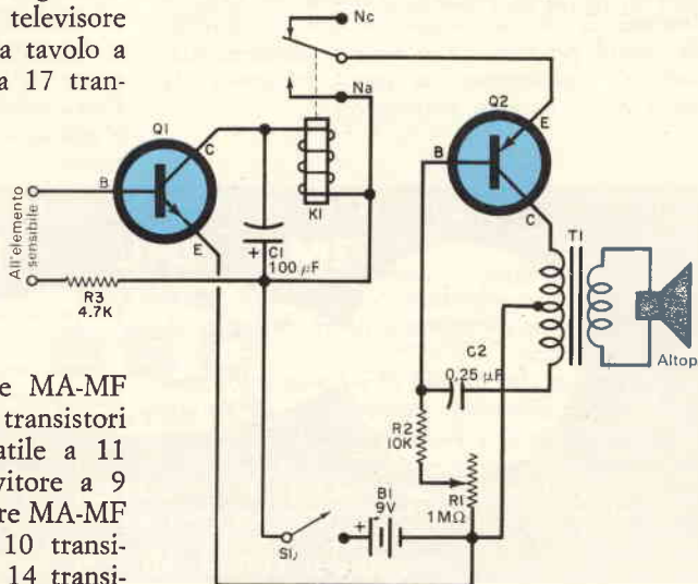
Fig. 1 - Questo sistema d'allarme anti-pioggia emette un suono udibile a distanza quando l'umidità si accumula sulla piastra sensibile.
