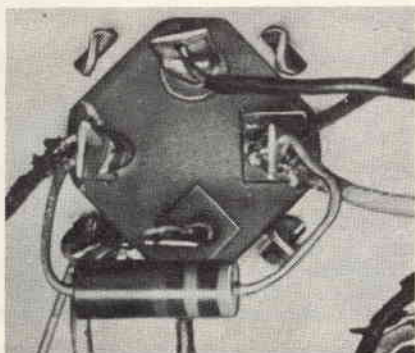
Montaggio di un condensatore di filtro con collegamenti lunghi. Tutti i terminali sono facilmente accessibili ed i diversi componenti sebbene sistemati vicini possono facilmente essere staccati.
