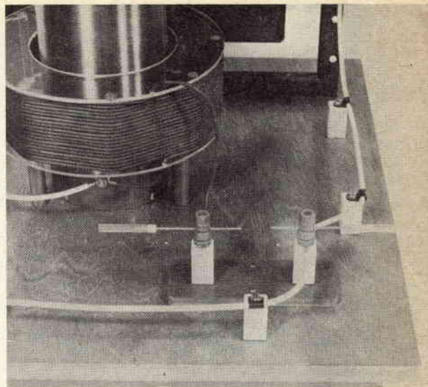
Lo spinterometro genera energia RF ed eccita la bobina. Gli elettrodi sono fatti con due fondini di rame montati su isolatori a colonna.
