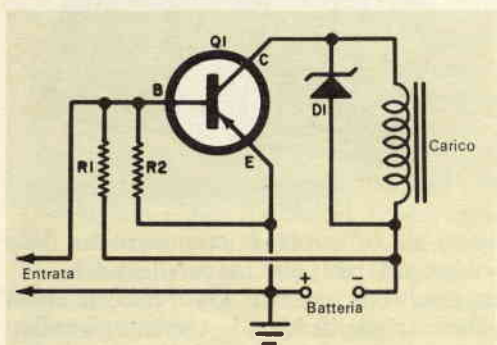
Fig. 2 - Tipico circuito per smorzare le eccessive tensioni transitorie. In esso è usato un diodo zener (D1) in parallelo al carico induttivo.
